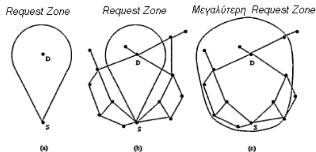
Σχήμα 3.6: Αιτούμενη Ζώνη (Request Zone): Μια ακμή συνδέει δύο κόμβους όταν είναι γειτονικοί
