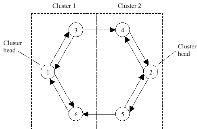
Σχήμα 3.4: Αμφίδρομα συνδεδεμένα clusters
