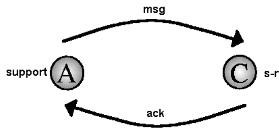
Σχήμα Ε.2: Το πρόβλημα της μετάδοσης από κόμβο υποστήριξης σε κόμβο sender-receiver
